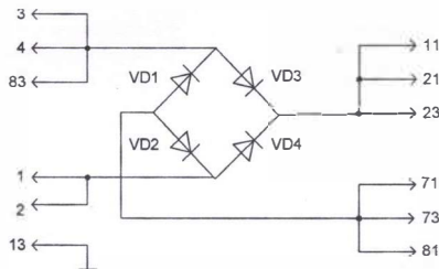
Схема электрическая принципиальная БВ-М
