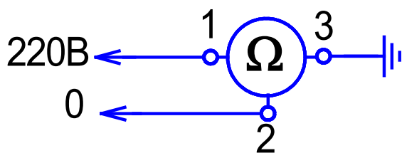
Рисунок 5.2 – Схема включения омметра
