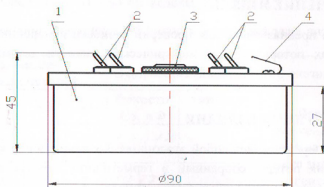
Рисунок 1 – Внешний вид ячейки
