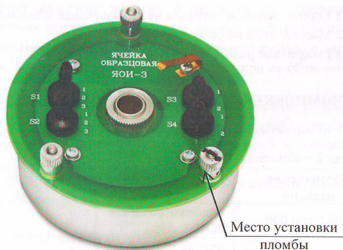
Рисунок 1 – Внешний вид ячейки
