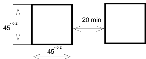
Рис.1. Вырез в щите для крепления регулятора.
