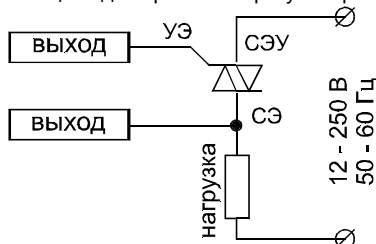
Рис.2. Схема подключения симисторов TC122-25, TC142-80.
