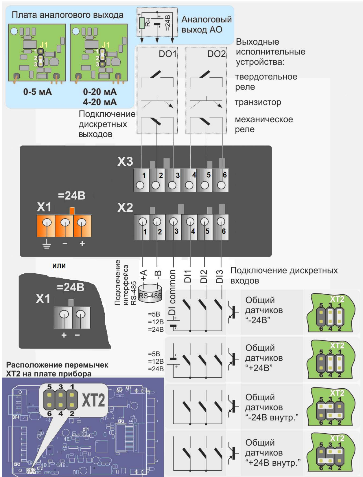
Рисунок Б.1.2 - Подключение внешних цепей счетчика МТЛ-32. Вид сзади. Исполнение на напряжении 24 В постоянного тока(такое же самое исполнение для счетчиков на 36 В постоянного тока)
