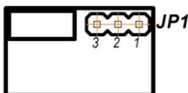
Рисунок 5.1 – Положение перемычек на модуле аналогового выхода
