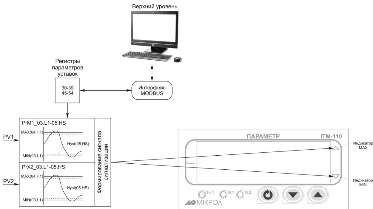
Рисунок 2.5 – Блок-схема блока сигнализации
